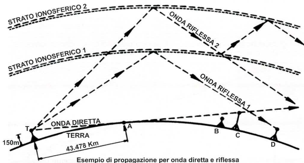
Esempio di propagazione per onda diretta e riflessa
